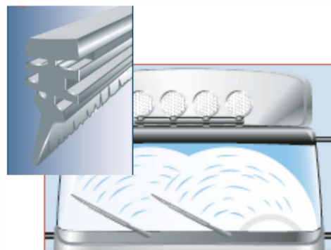
Растрескивание щеток приводит к появлению полос
