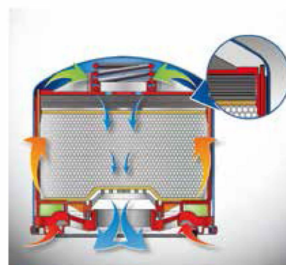
Масляный фильтр расположен над поглотителем влаги
